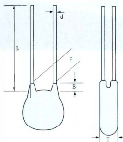
capacitor cerâmico
