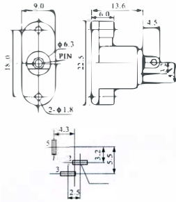
DC-019 J4
