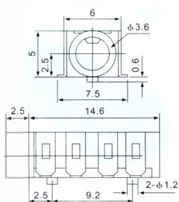
PJ-3020B
